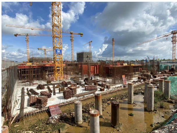
6#栋筏板施工
